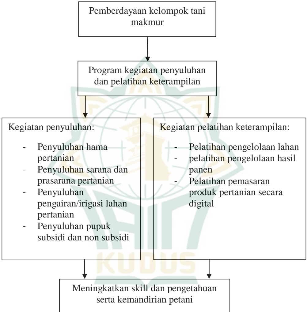
Gambar 2 .1. Kerangka Berfikir
