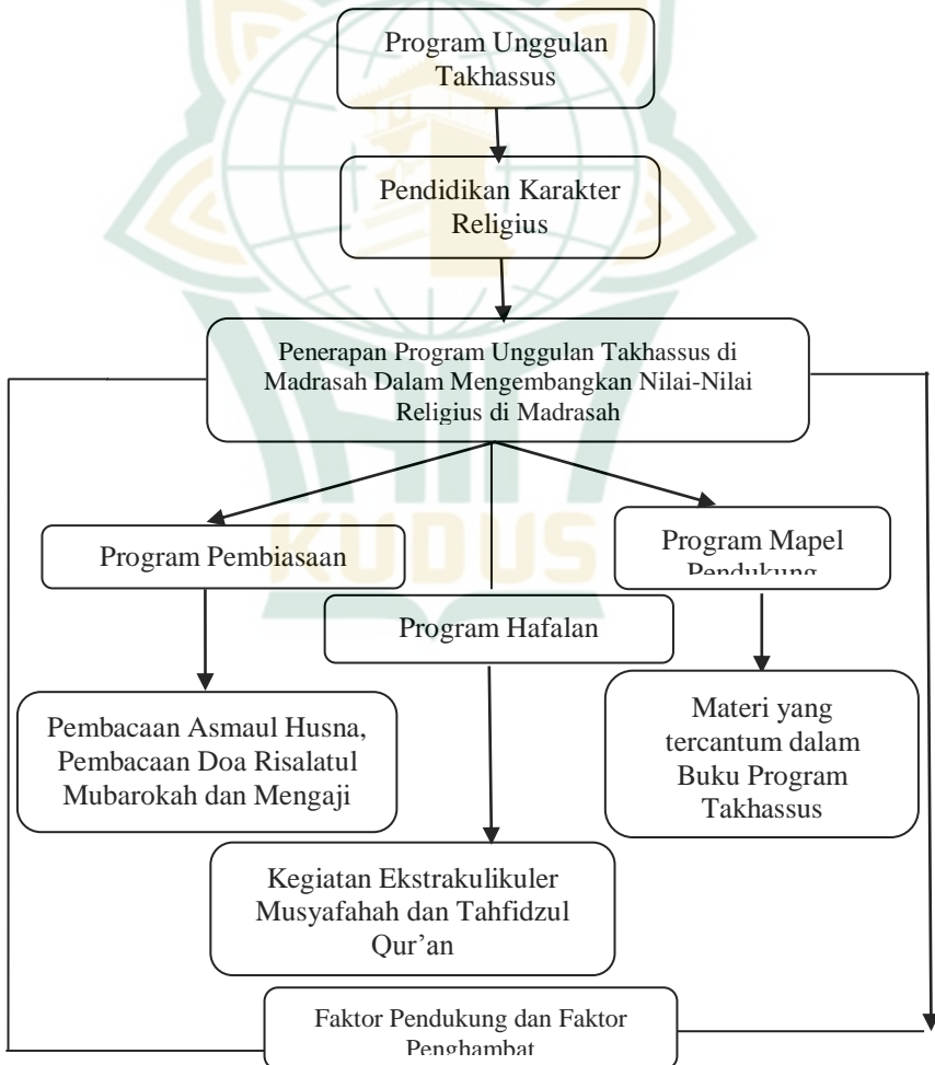
Gambar 2.3 Kerangka Berpikir
