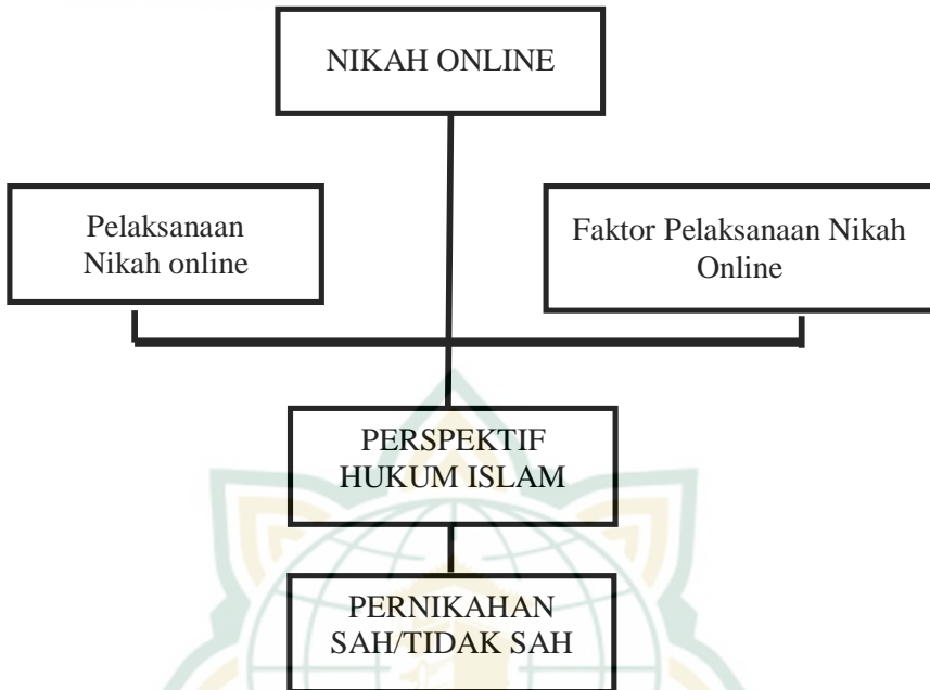
Gambar 2.1 Kerangka Pikir
