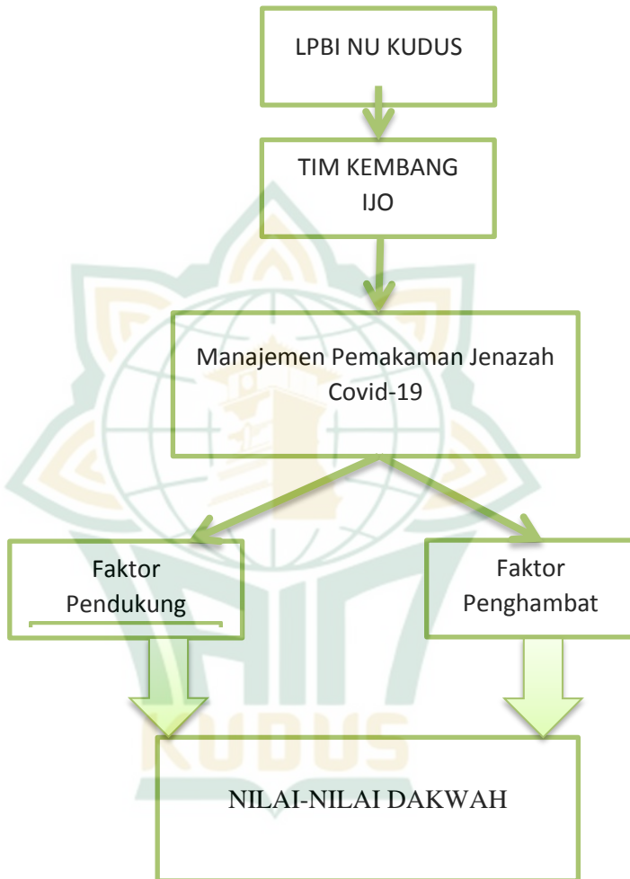
Gambar 2.1 Kerangka Berpikir
