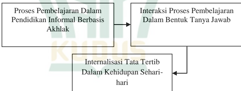
Gambar 3.1. Penyajian Data
