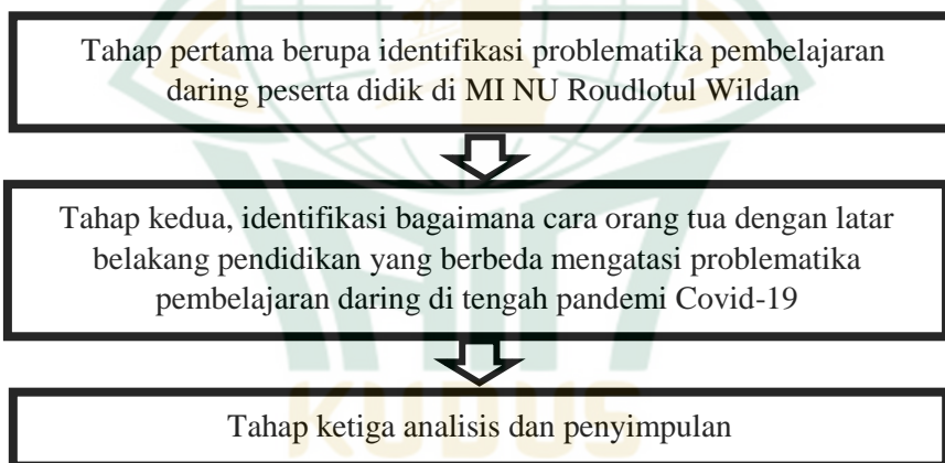
Gambar 3.1. Langkah-langkah Penelitian
