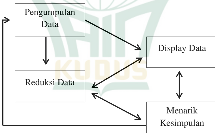
Gambar 3.1 Teknik Analisis
