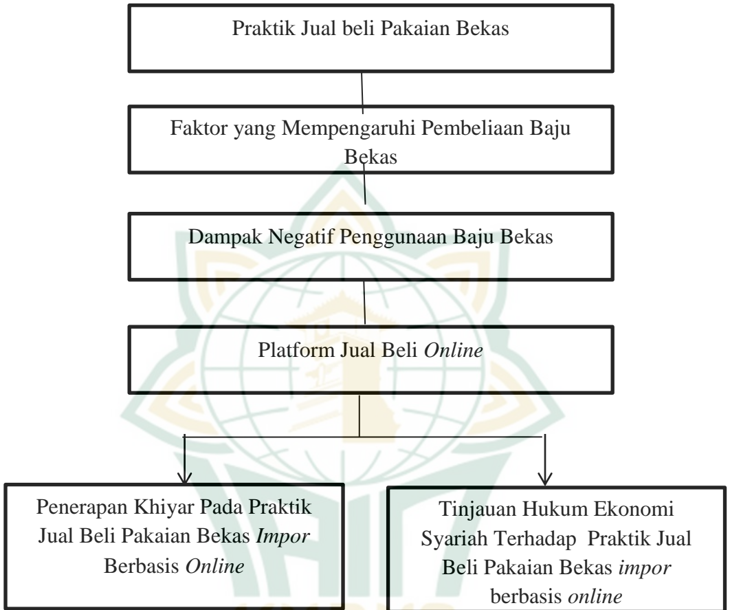
Gambar 2.3 Kerangka Berpikir
