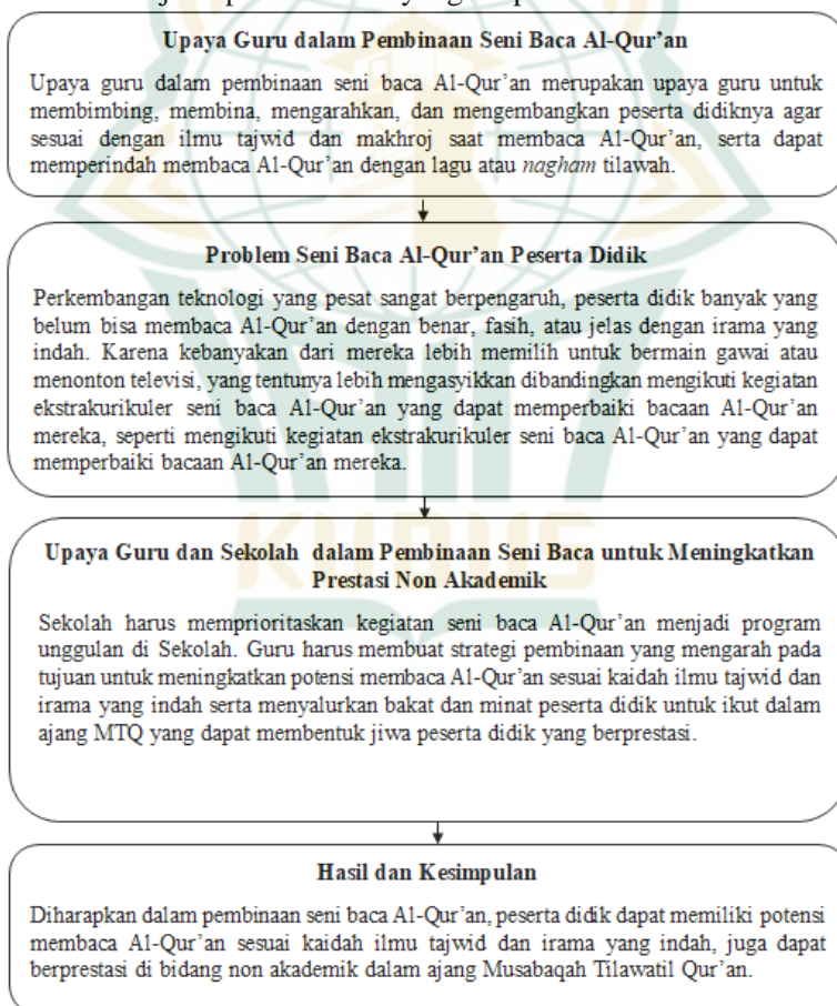
Gambar 2.1 Kerangka Berpikir
